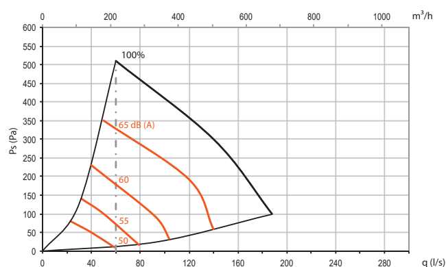
Lydeffektnivå til avtrekkslufterkanal/uteluftkanal
