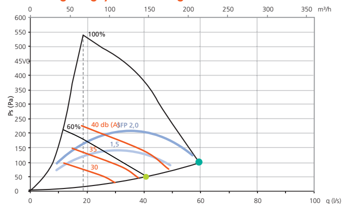
Luftmengde og lydnivå til omgivelsene
