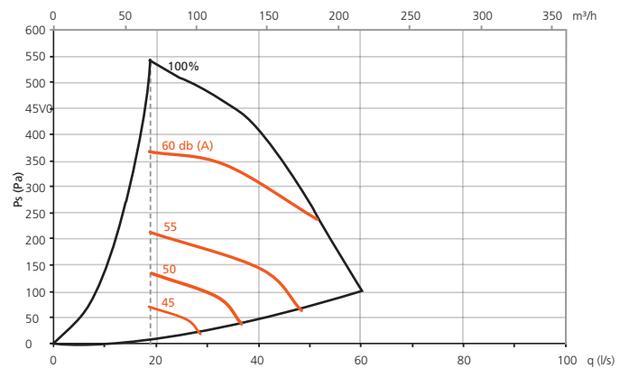
Lydeffektnivå til avtrekksluftkanal
