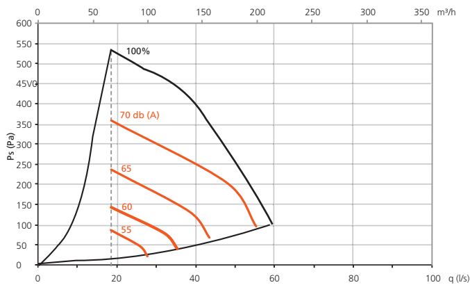
Lydeffektnivå til avkastkanal
