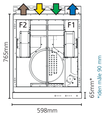
Kjøkkenhette JAZZ *iden måle 90 mm
