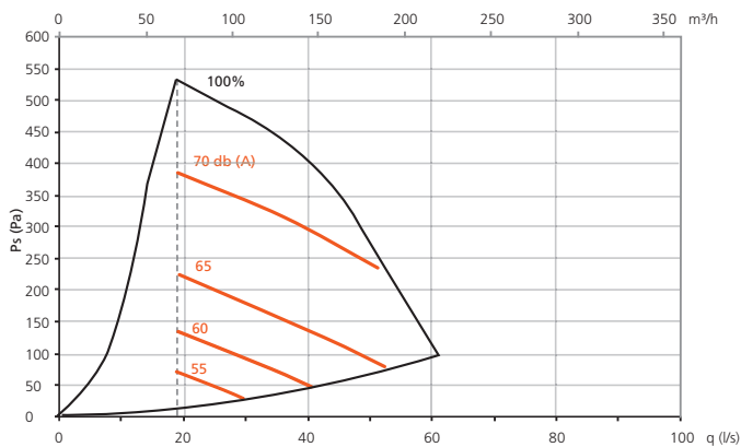
Lydeffektnivå til tilluftskanal
